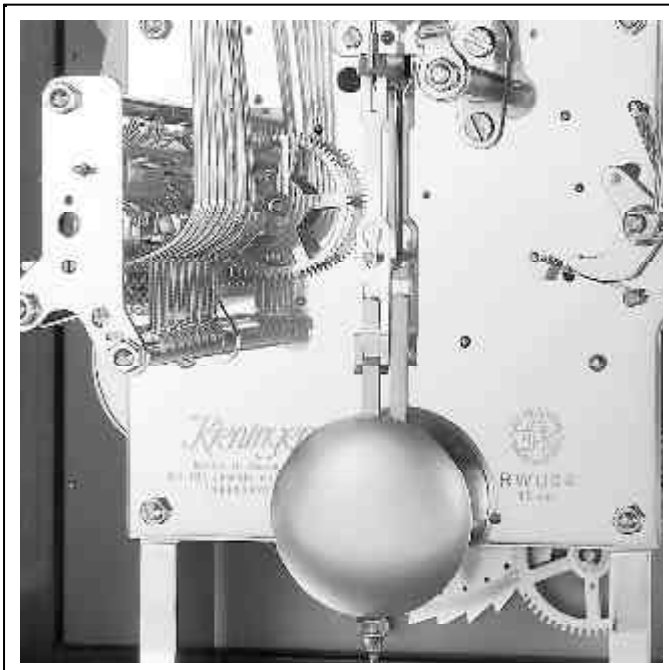
Bild 2 / Picture 2 / Figure 2 / Ilustración 2 Pendelfeder, Pendelverlängerung und Weiserstift Suspension spring, pendulum extension and verge pin Ressort, support et indicateur du pendule Resorte de suspensión, alargadera de la péndola y perno de aguja
